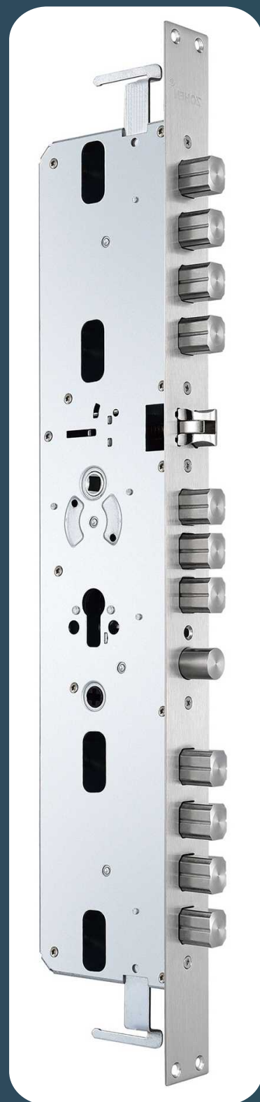
CSA600E (60/68) Size: 40*600*102mm
