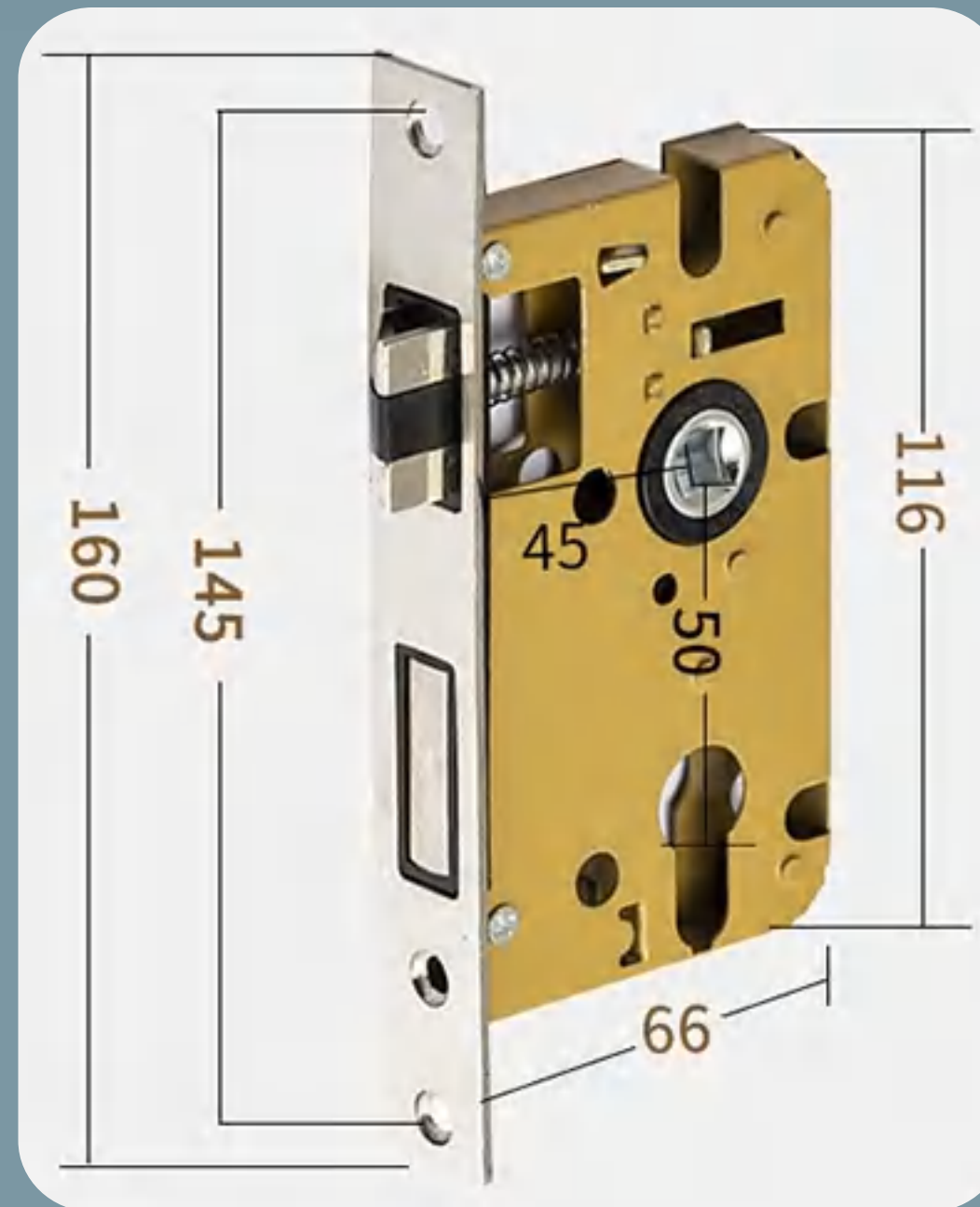
CSA5045 Silent lock body
