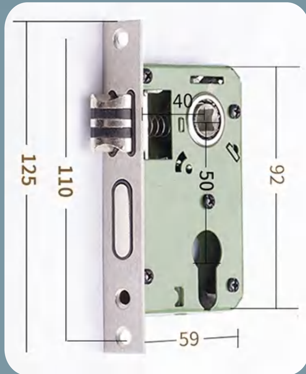
CSA5040 Silent lock body
