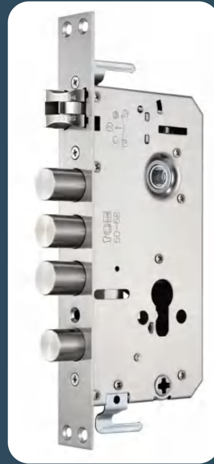
CSA802 Size: 30*240*92mm
