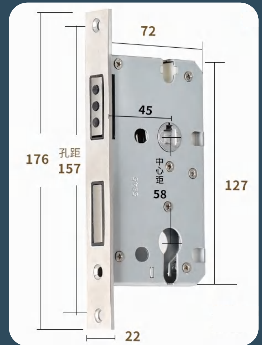
CSA5845 Magnetic lock body
