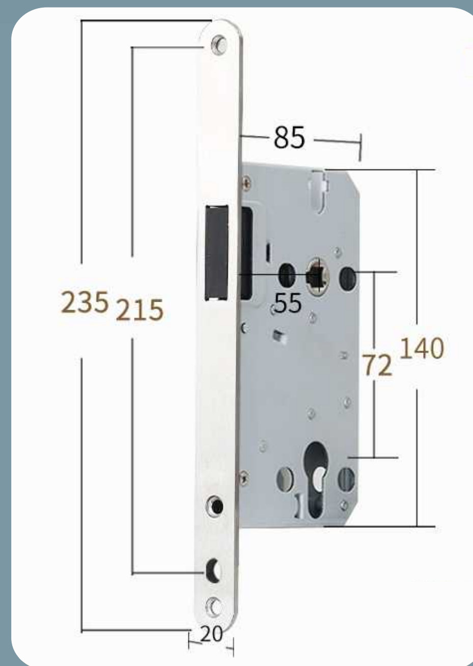
CSA7255 Magnetic lock body
