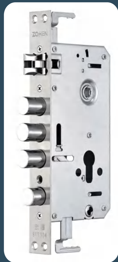
CSA836 Size: 30*240*92mm
