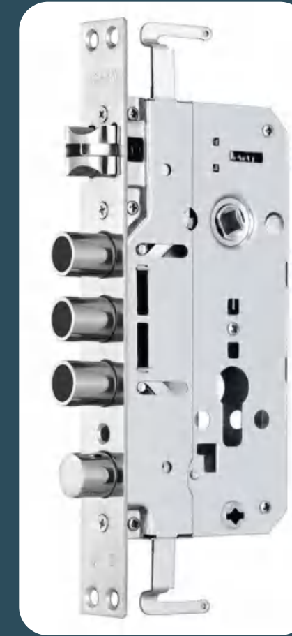
CSA806 Size: 30*240*89mm
