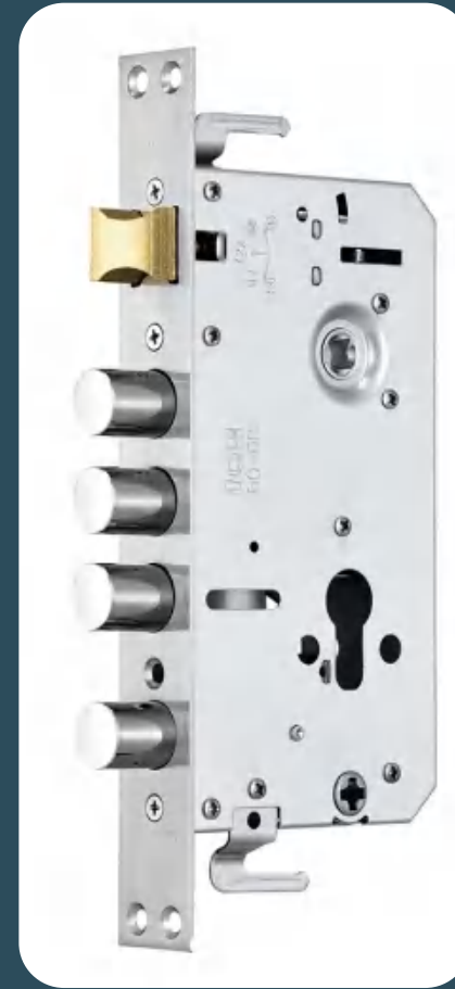
CSA802A Size: 30*240*92mm
